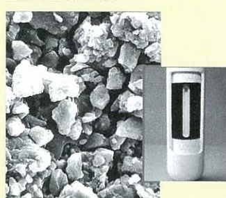
Stage 2 系統二： Pressed-Carbon Block Magnified 1000x. 放大1000倍的系統二濾材
