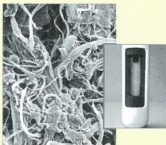
Stage 1 系統一： Multi-Composite Media Magnified 250x. 放大250倍的系統一濾材
